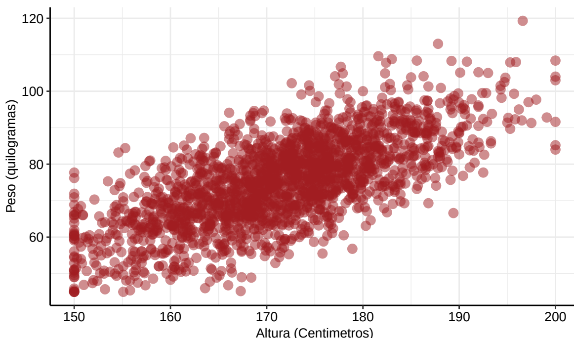
Figura 2: Gráfico de dispersão da altura (Centímetros) pelo peso (quilogramas)
