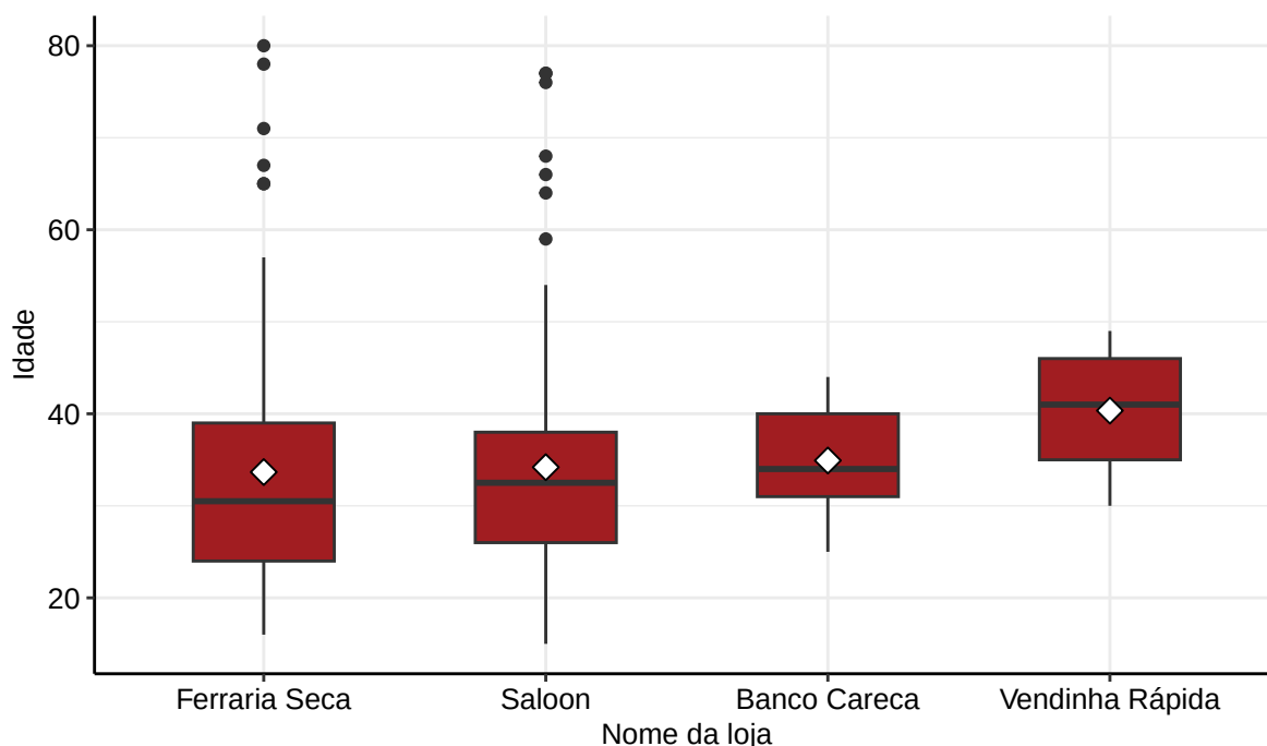
Figura 3: Boxplot bivariado da idade do cliente por Nome da loja em Ambar Seco
