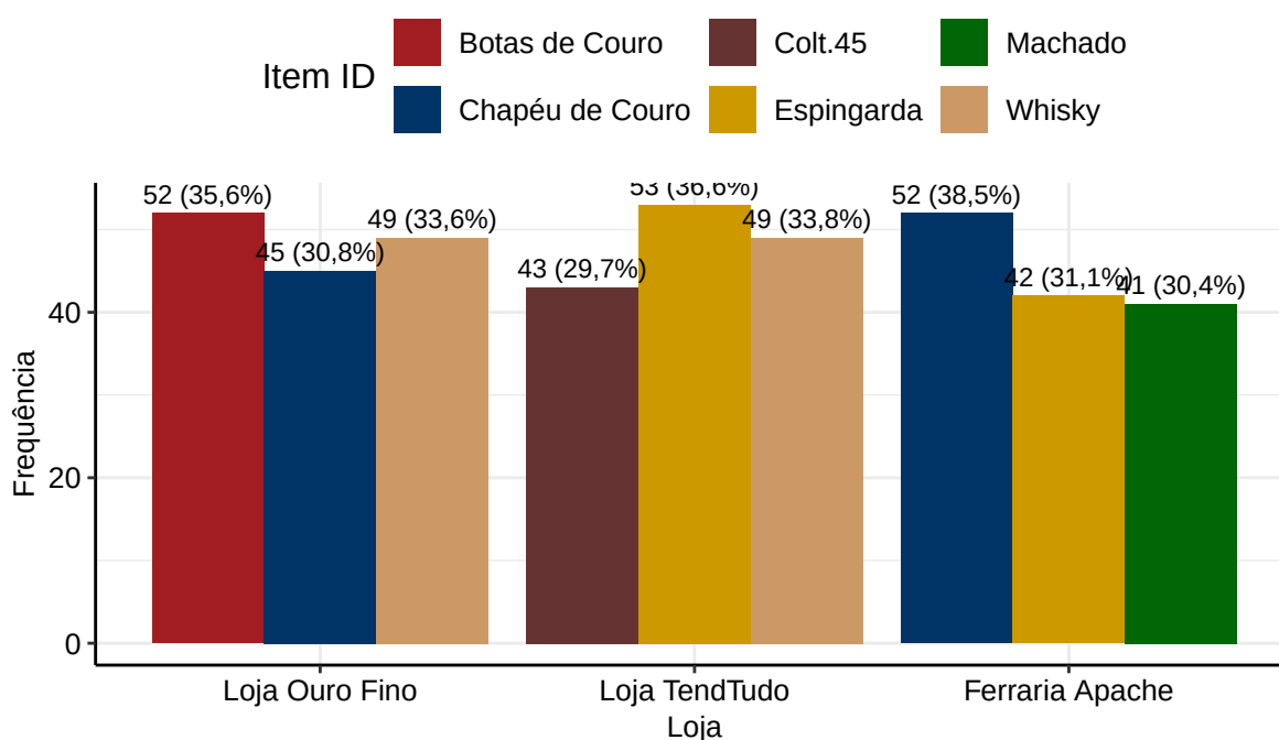
Figura 4: Gráfico de colunas da loja pelo frequência de vendas
